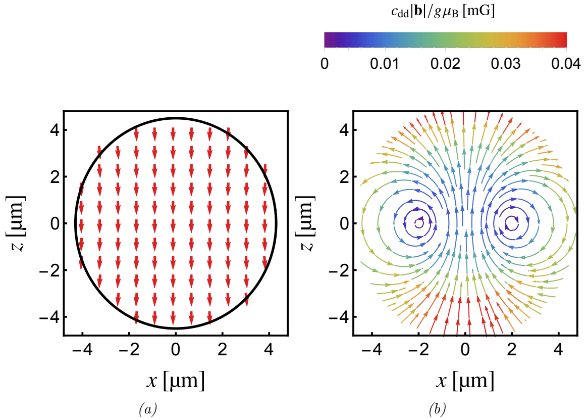
FIGURE 1.9 – État fondamental pour c_{dd} \neq 0 et p/g\mu_B = 0.24 \text{ mG} . (a) : Projections du vecteur \mathbf{f} , dans le plan xz . (b) : Projections du champ dipolaire \mathbf{b} , dans le plan xz . Le code couleur indique c_{dd}|\mathbf{b}| . Calculs réalisés pour un condensat de ^{52}\text{Cr} avec N = 40 \times 10^3 et \omega/2\pi = 260 \text{ Hz} .
