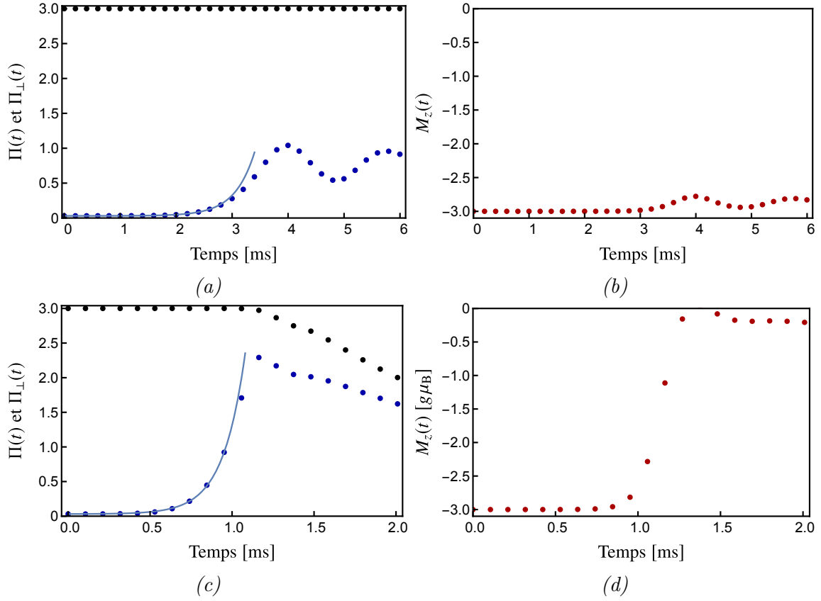
FIGURE 3.2 – Évolution de M_z , \Pi et \Pi_\perp pour p = 0.9 \times p_{\text{add}} ((a) et (b)) et p = 0.0 \times p_{\text{add}} ((c) et (d)). La courbe pleine est obtenue à partir de (3.10). (a) : \Pi_\perp(0) \simeq 0.03 , \lambda = 0.6 \times 10^{-4} et \hbar/\gamma \simeq 2.2 ms. Les données sont fittées jusqu'à t \simeq 3.4 ms (c) : \Pi_\perp(0) \simeq 0.03 , \lambda = 0.7 \times 10^{-3} et \hbar/\gamma \simeq 0.85 ms. Les données sont fittées jusqu'à t \simeq 1.2 ms. Ces calculs ont été réalisés pour un condensat de ^{52}\text{Cr} uniforme de densité n = 1.54 \times 10^{21} \text{m}^{-3} .
