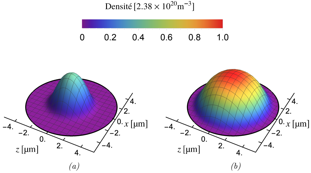
FIGURE 1.6 – État fondamental pour c_{dd} = 0 et p/g\mu_B = 0.12 \text{ mG} . Les figures (a) et (b) représentent, dans l'ordre, des coupes des densités n_2 et n_{-3} dans le plan xz . Calculs réalisés pour un condensat de ^{52}\text{Cr} avec N = 40 \times 10^3 et \omega/2\pi = 260 \text{ Hz} .
