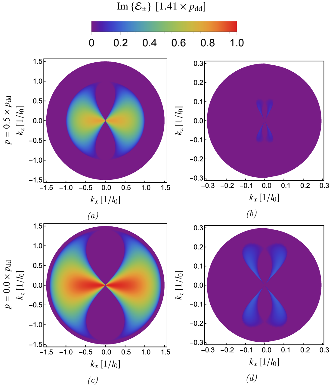
FIGURE 2.1 – Parties imaginaires des spectres énergétiques \mathcal{E}_{\pm} dans le plan k_x k_z . Pour certaines valeurs de k_x et k_z seule l'énergie \mathcal{E}_{-} est imaginaire : \text{Im}\{\mathcal{E}_{+}\} = 0 et \text{Im}\{\mathcal{E}_{-}\} > 0 . Pour d'autres valeurs de k_x et k_y les énergies \mathcal{E}_{\pm} sont complexes conjuguées : \text{Im}\{\mathcal{E}_{+}\} > 0 et \text{Im}\{\mathcal{E}_{-}\} = -\text{Im}\{\mathcal{E}_{+}\} . Pour la clarté, nous avons représenté uniquement les valeurs positives de \text{Im}\{\mathcal{E}_{\pm}\} . (a) et (c) : partie imaginaire positive de \mathcal{E}_{\mathbf{k},-} , respectivement pour p = 0.5 \times p_{\text{dd}} et p = 0.0 \times p_{\text{dd}} . (b) et (d) : partie imaginaire de \mathcal{E}_{+} , respectivement pour p = 0.5 \times p_{\text{dd}} et p = 0.0 \times p_{\text{dd}} . Ces calculs sont réalisés pour un condensat de ^{52}\text{Cr} uniforme de densité n = 1.54 \times 10^{21} \text{m}^{-3} . L'unité d'énergie est p_{\text{dd}} \simeq 1 \text{ Hz} et l'unité de longueur est l_0 = \sqrt{\hbar^2 / 2M p_{\text{dd}}} \simeq 0.44 \mu\text{m} .
