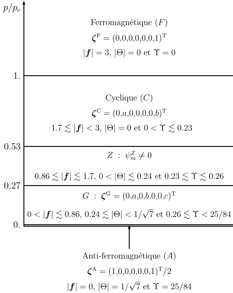
FIGURE 1.3 – Diagramme de phase d'un condensat uniforme de ^{52}\text{Cr} en fonction de p/p_c . Le champ magnétique critique p_c est définie par (1.137).
