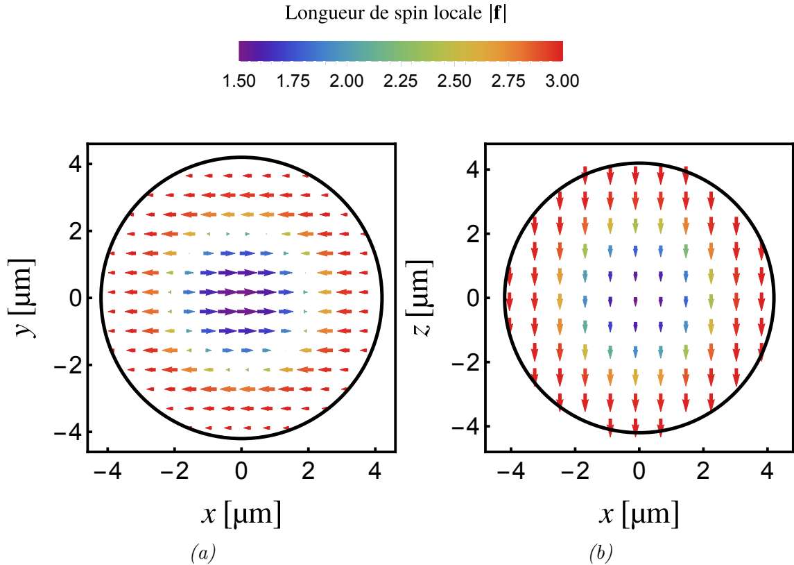
FIGURE 1.7 – État fondamental pour c_{dd} = 0 et p/g\mu_B = 0.12 \text{ mG} . Les figures (a) et (b) représentent, dans l'ordre, les projections du vecteur \mathbf{f} , dans les plans xy et xz . Le code couleur indique |\mathbf{f}| . La longueur des flèches indique la longueur des spins dans les plans xy et xz . Calculs réalisés pour un condensat de ^{52}\text{Cr} avec N = 40 \times 10^3 et \omega/2\pi = 260 \text{ Hz} .
