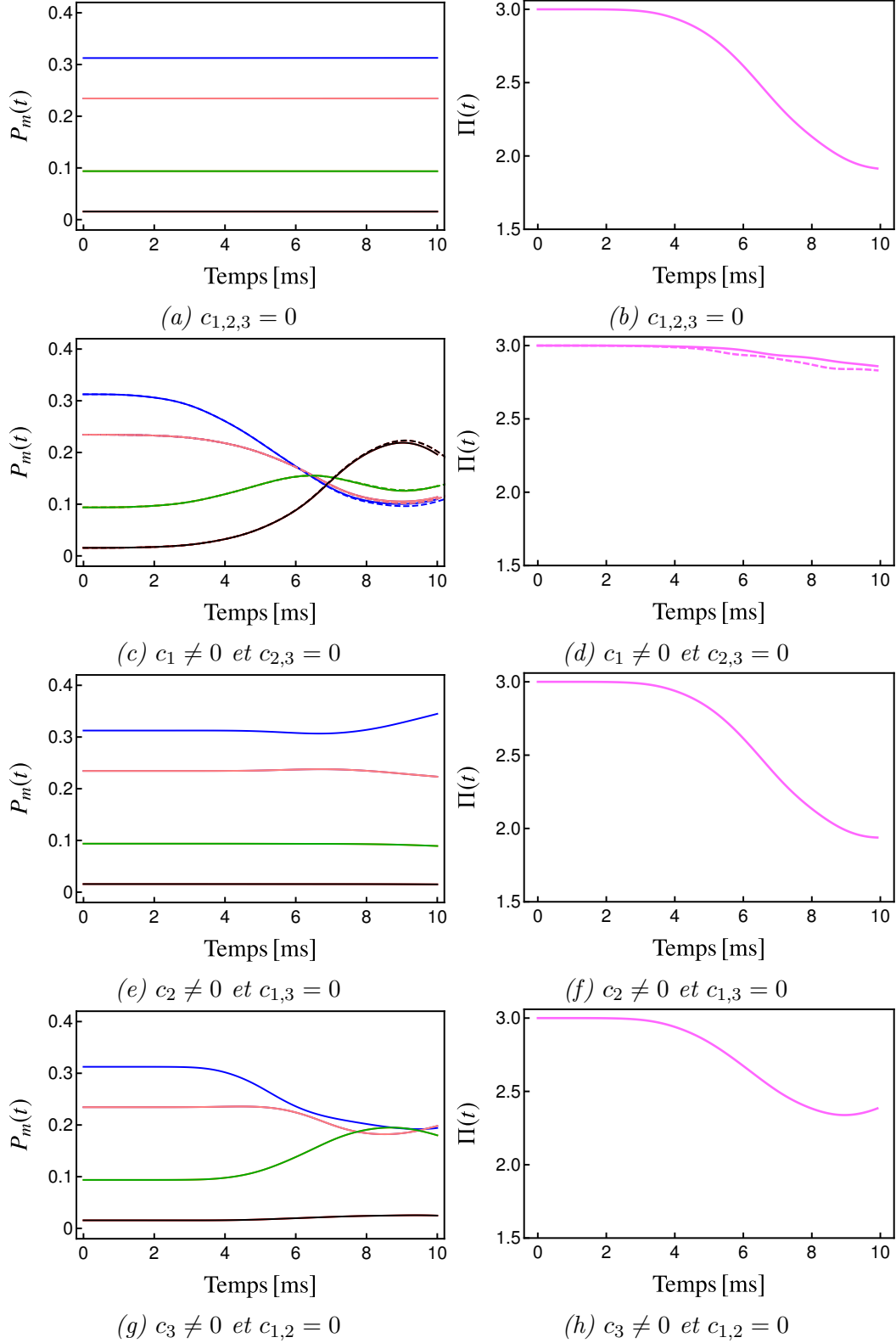
FIGURE C.1 – Évolution des P_m et \Pi . Code couleur des P_m : m = \pm 3 (noir), m = \pm 2 (vert), m = \pm 1 (rose) et m = 0 (bleu). Pour ces simulations, nous avons pris en compte les valeurs des gradients \gamma_{zx} = 2.55 \text{ mG cm}^{-1} , \gamma_{zy} = 51 \text{ mG cm}^{-1} , \gamma_{zz} = -3.22 \text{ mG cm}^{-1} , et q = 6 \text{ Hz} . Calculs réalisés pour un condensat de ^{52}\text{Cr} avec N_{\text{tot}}(0) = 38 \times 10^3 dans un piège harmonique de fréquences \omega_x/2\pi = 298 \text{ Hz} , \omega_y/2\pi = 245 \text{ Hz} et \omega_z/2\pi = 210 \text{ Hz} .
